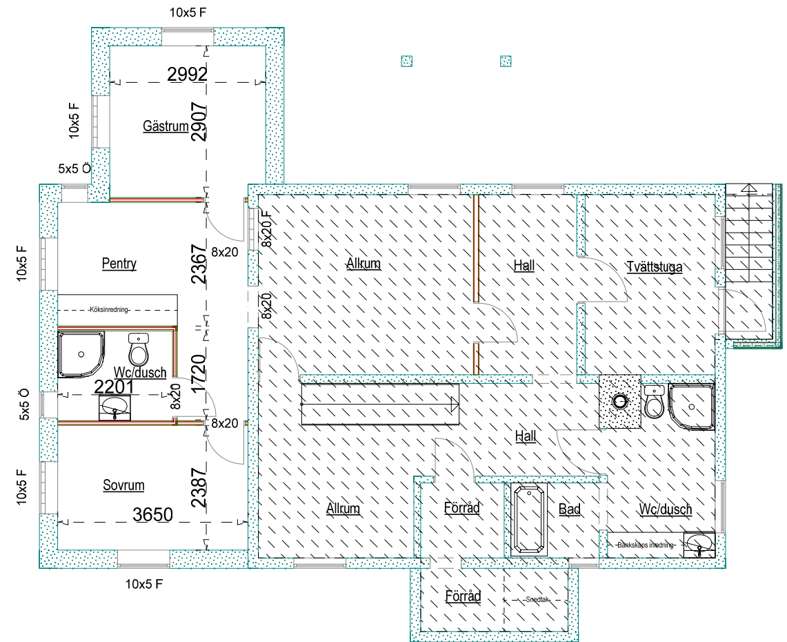
Källarplan
