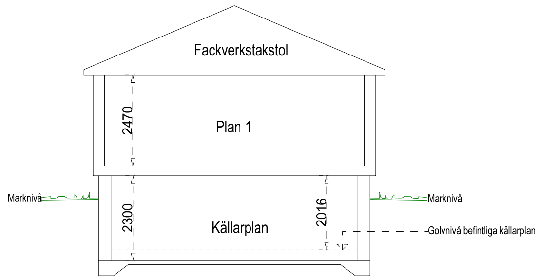
Sektion A-A
